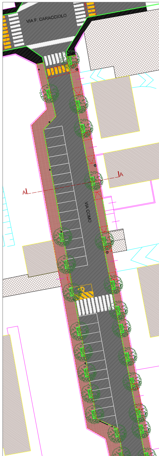
PLANIMETRIA OPERE SOPRASUOLO nord scala 1:200
